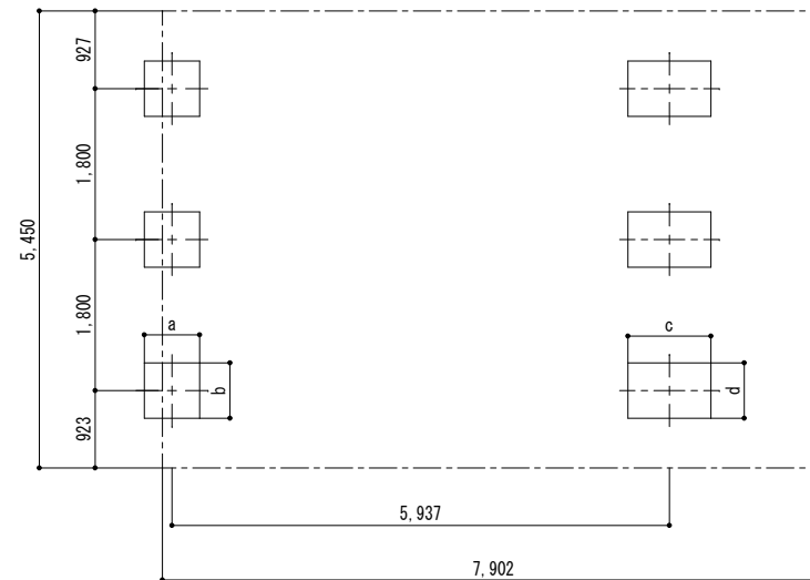
■ 基礎配置図
